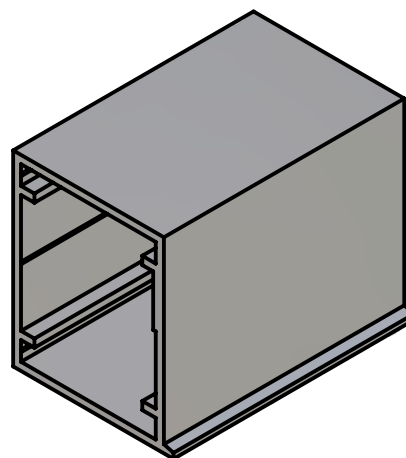
detail kaderprofiel
