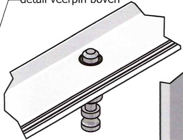
detail tussenprofiel
